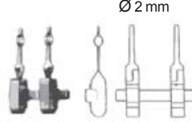
BIEMER-MULLER S 014.00 Çene uzunluğu / Length of jaws 9 mm Açıklık / Opening 5 mm Kapanma kuvveti / closing force 25-30 gr.
