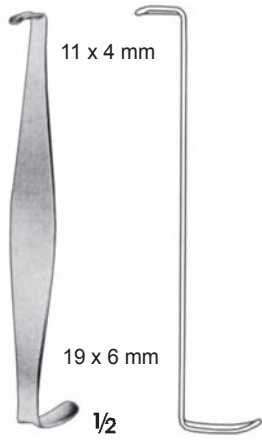
CRILE K 300.00 11 cm
