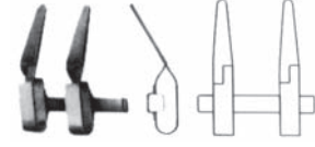
BIEMER-MULLER S 012.00 Çene uzunluğu/Lenght of jaws.9 mm Açıklık/Opening 5 mm Kapanma Kuvveti/Closing force 25-30 gr.
